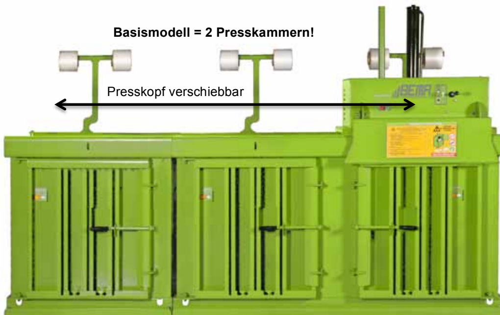
Abb. Modell mit 3 Kammern (Optional)
